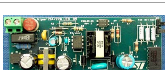
STEVAL-ILL006V1
