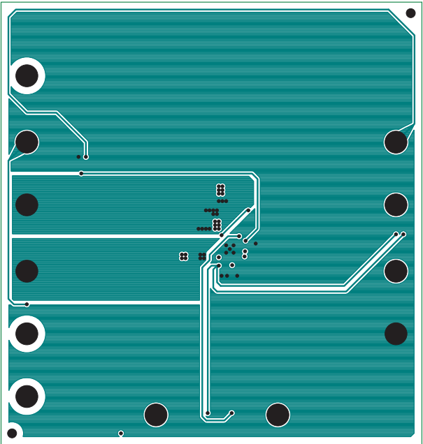
Inner Layer 2
