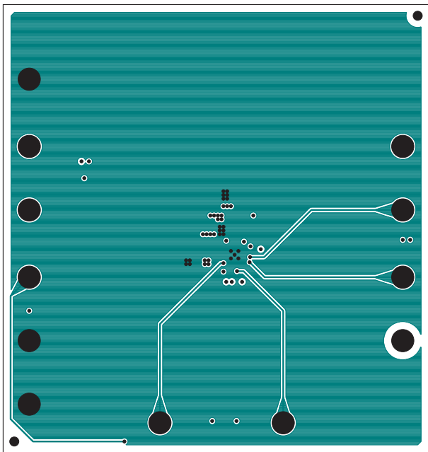
Inner Layer 3
