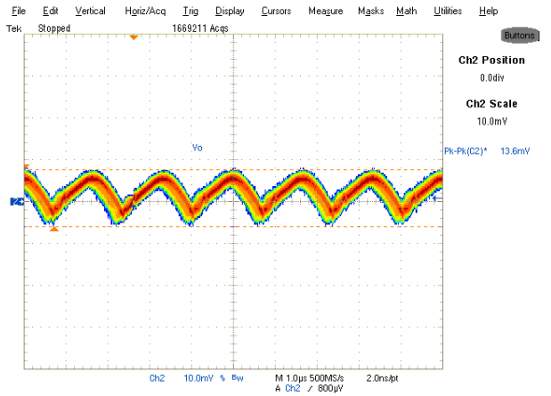
Fig. 20. Output Voltage Ripple, 4A load Ch 2 : V_o
