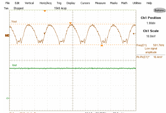
Fig. 10: Output Voltage Ripple, 12A load Ch 1 : V out , Ch 4 : I out
