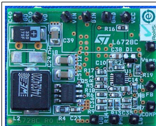
STEVAL-ISA038V1
