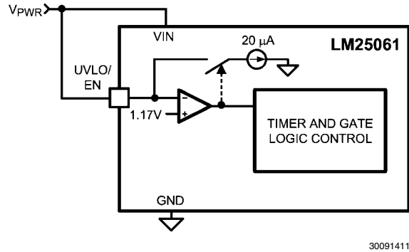
FIGURE 6. UVLO = POR
