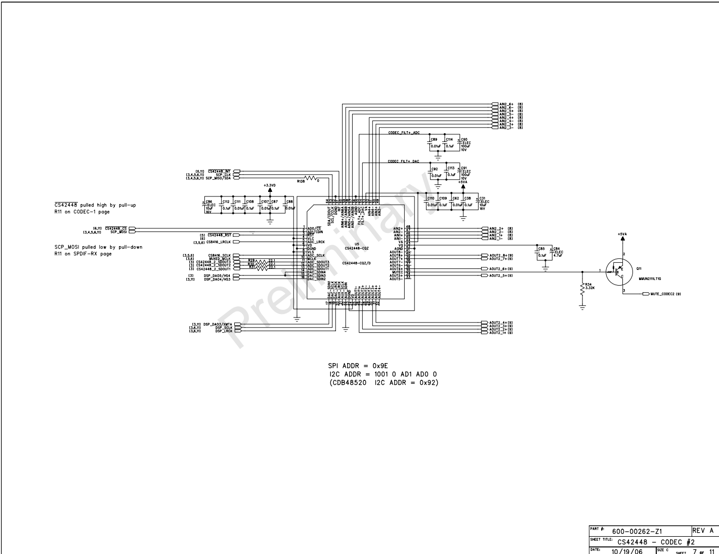
Figure A-7. Codec #2 (CS42448)
