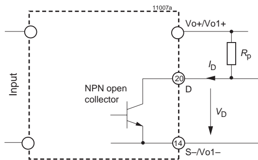
Fig. 39 Option D5 – DD: NPN output, V_{o1} \leq 40 V, I_D \leq 20 mA
