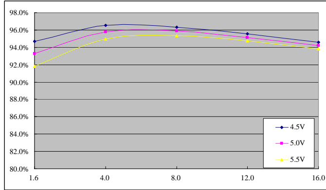
Vo=3.3 V
