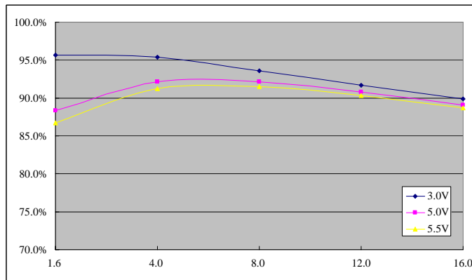
Vo=1.8 V
