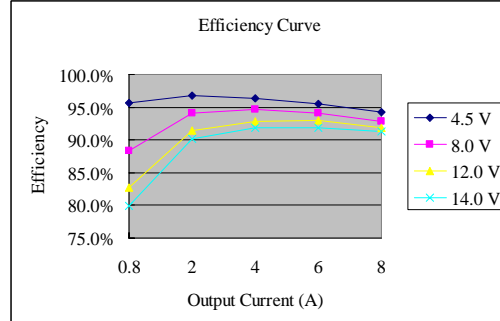
Vo=3.3 V
