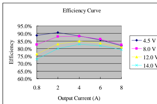
Vo=0.9 V
