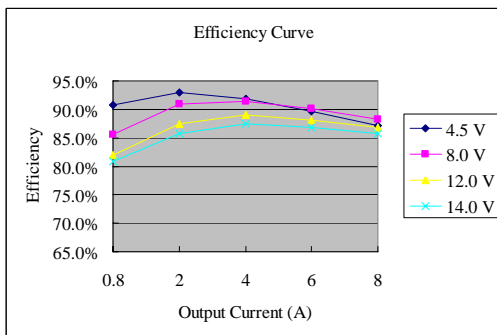
Vo=1.5 V
