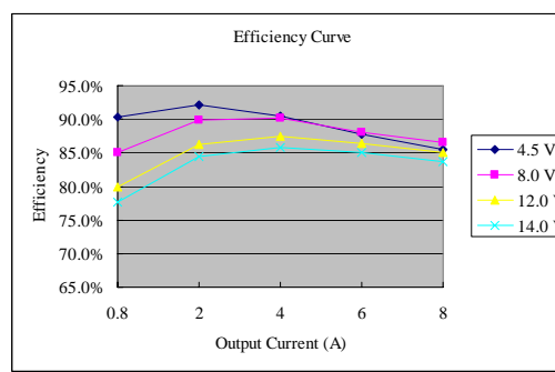
Vo=1.2 V
