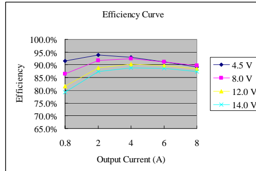
Vo=1.8 V
