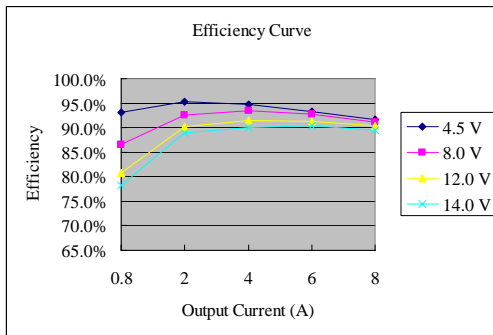
Vo=2.5 V
