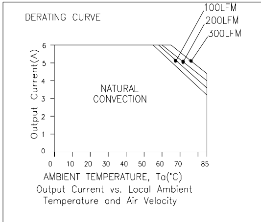
Vin=5.0 V, Vo=3.3 V
