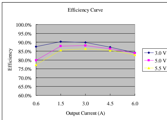
Vo=1.2 V
