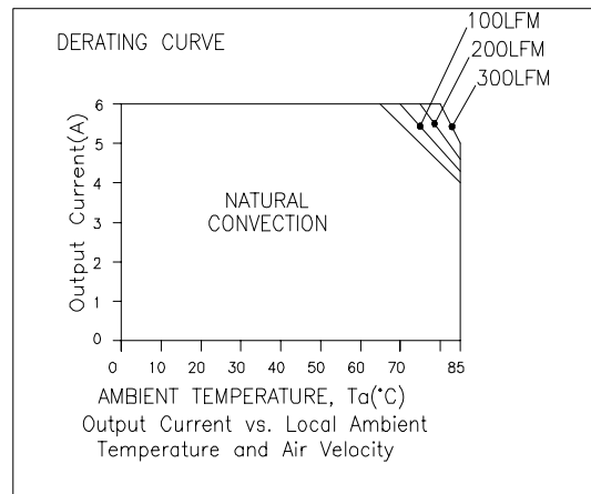
Vin=3.3 V, Vo=0.75 V
