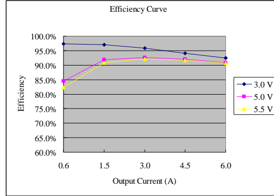
Vo=2.5 V
