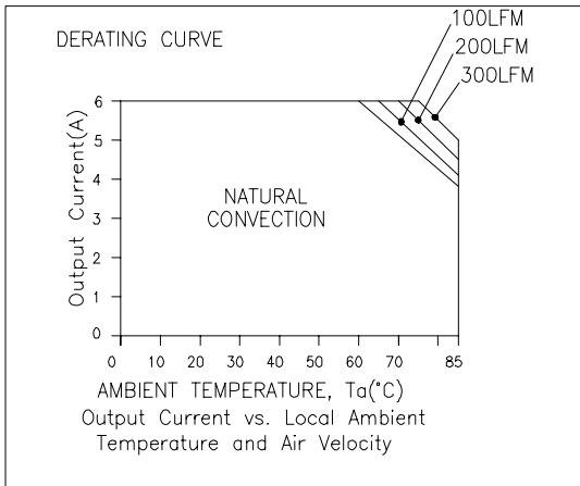
Vin=3.3 V, Vo=2.5 V
