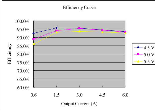
Vo=3.3 V
