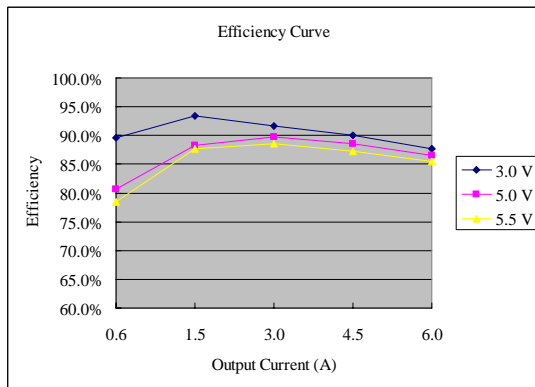
Vo=1.8 V
