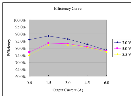
Vo=0.7525 V
