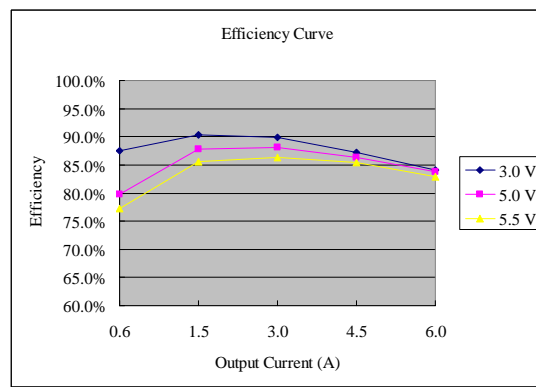
Vo=1.5 V
