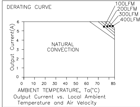
V_{in}=12\text{ V}, V_o=0.75\text{ V}
