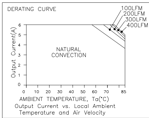
V_{in}=12\text{ V}, V_o=2.5\text{ V}
