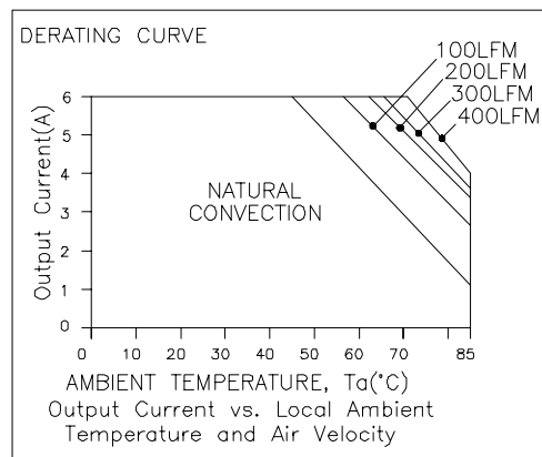
V_{in}=12\text{ V}, V_o=5.0\text{ V}
