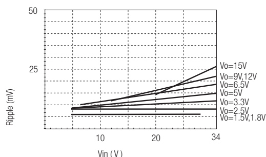
Ripple Vs Vin (Full Load)
