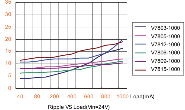
Ripple(mV)
