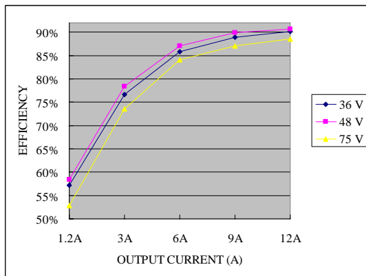
Vo=5.0 V
