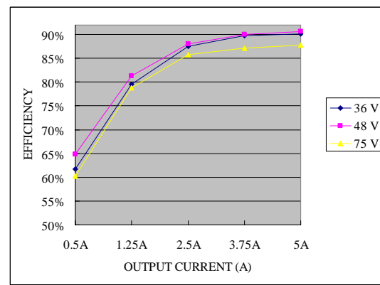
Vo=12 V
