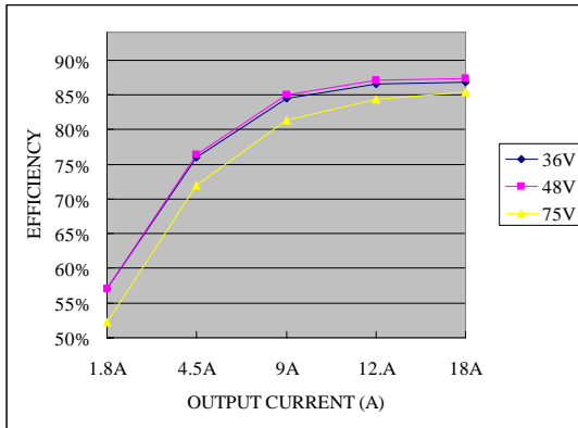
Vo=2.5 V
