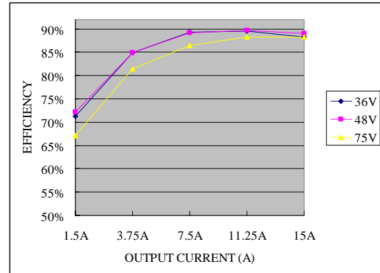
Vo=3.3 V
