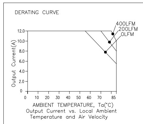
Vo=5 V
