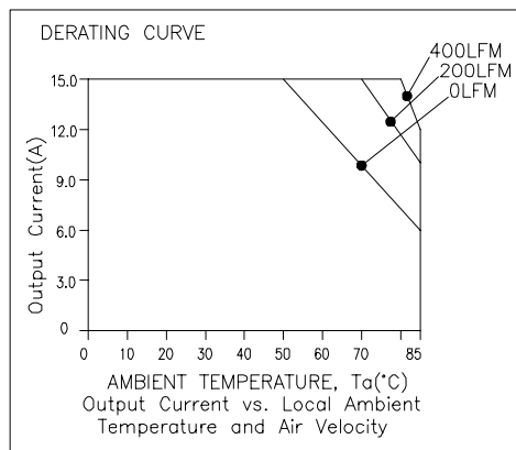
Vo=3.3 V
