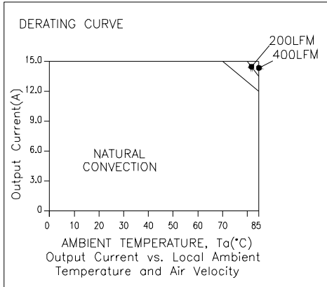
Vo=1.2 V
