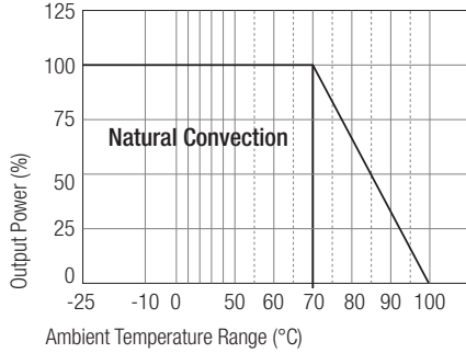
RP10-2405DEW
