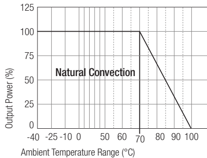
RP10-2405DEW/M2
