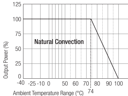
RP10-2405DEW/M2
