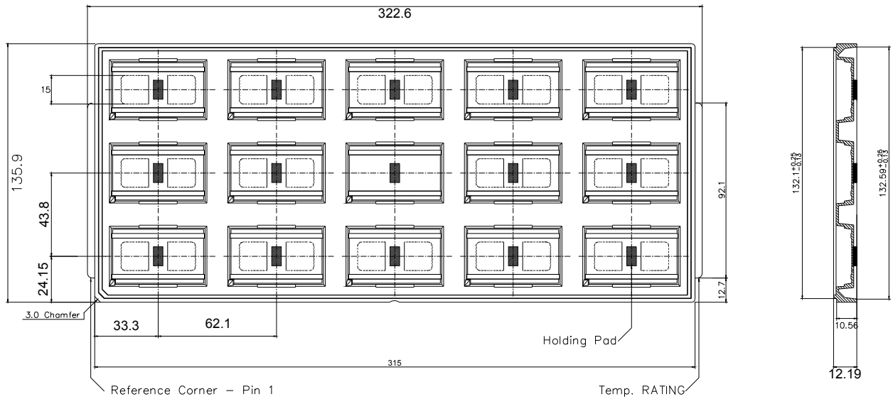
JEDEC TRAY
