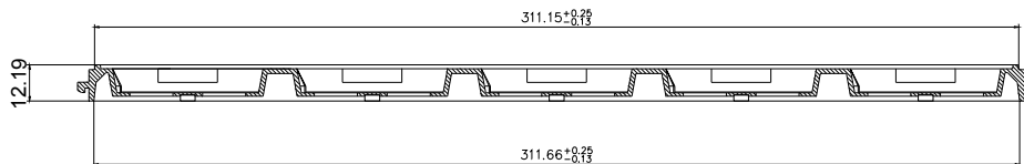
JEDEC TRAY
