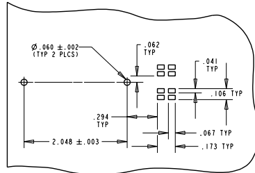
SOLDER PAD/HOLES LAYOUT SCALE: 2:0
