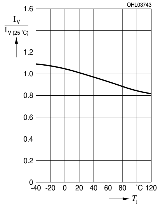
Relative Lichtstärke 2) Seite 19 Relative Luminous Intensity 2) page 19 I_V/I_V(25\text{ °C}) = f(T_j); I_F = 1\text{ A}; \text{LE T G3W}
