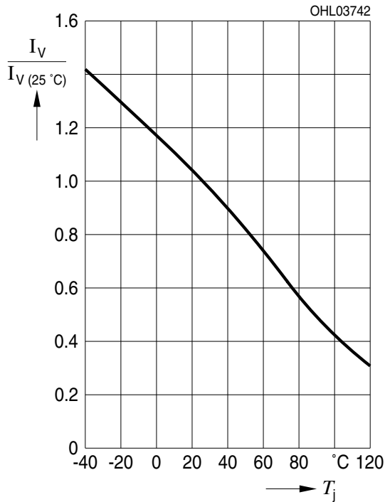
Relative Lichtstärke 2) Seite 19 Relative Luminous Intensity 2) page 19 I_V/I_V(25\text{ °C}) = f(T_j); I_F = 1\text{ A}; \text{LE B G3W}
