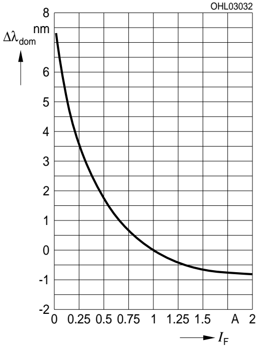
Dominante Wellenlänge 2) Seite 16 Dominant Wavelength 2) page 16 LB, \lambda_{\text{dom}} = f(I_F); T_{\text{board}} = 25\text{ °C}
