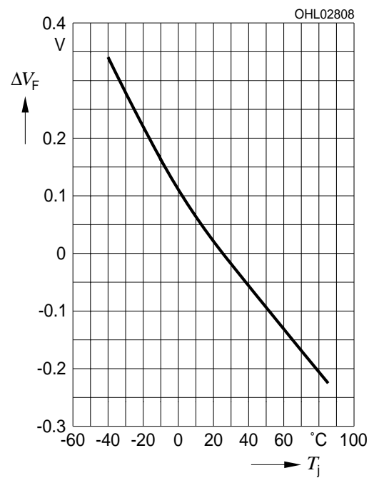
Relative Vorwärtsspannung 2) Seite 17 Relative Forward Voltage 2) page 17 \Delta V_F = V_F - V_{F(25\text{ °C})} = f(T_j); I_F = 1000\text{ mA (blue)}
