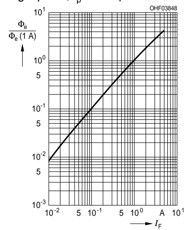
Relativer Gesamtstrahlungsfluss Relative Total Radiant Flux \Phi_e / \Phi_e(1\text{ A}) = f(I_F), T_B = 25\text{ °C}, Single pulse, t_p = 100\ \mu\text{s}
