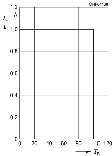
Max. zulässiger Durchlassstrom Max. Permissible Forward Current I_F = f(T_B), R_{thJB} = 3\ \text{K/W}
