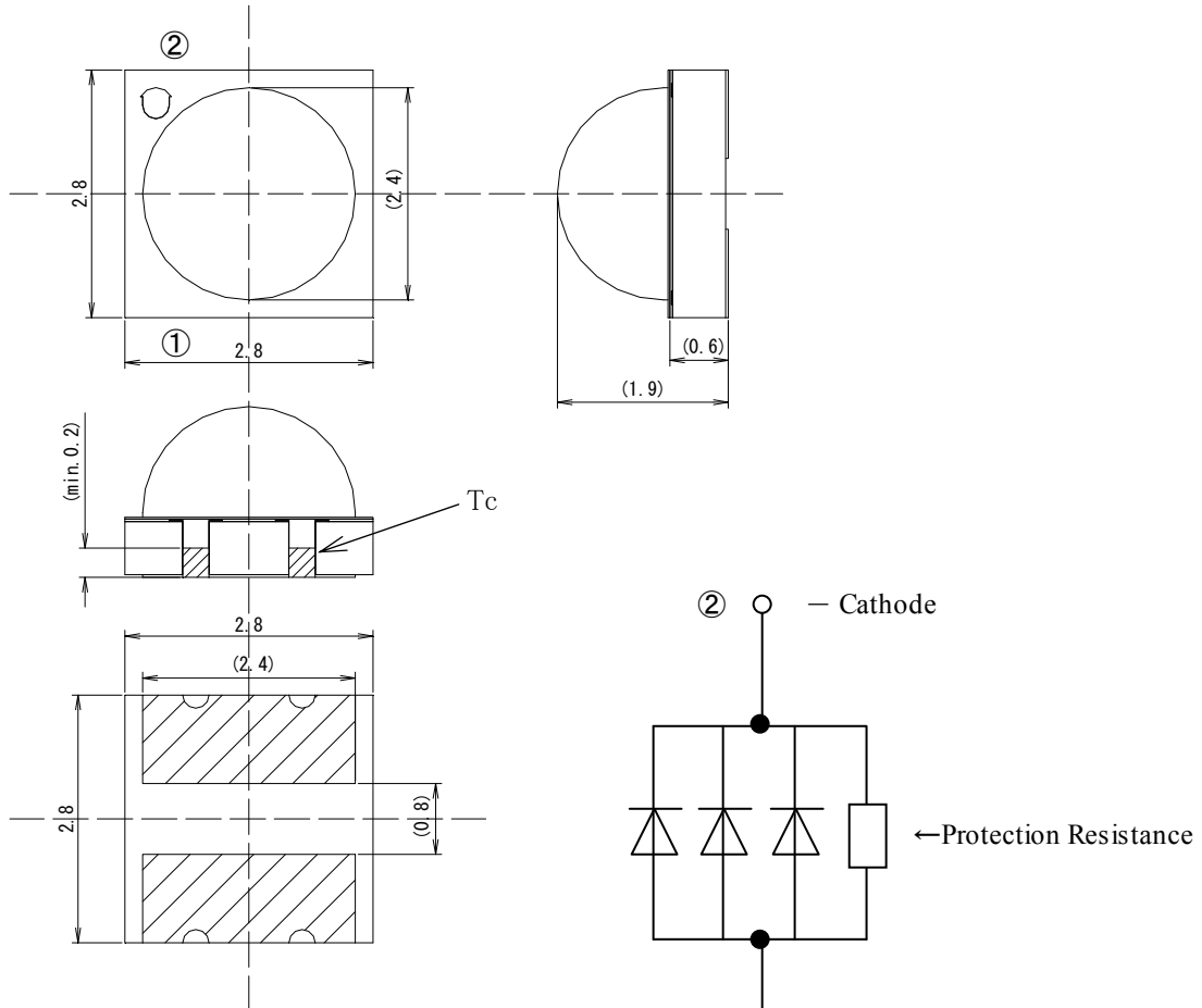
① + Anode ② - Cathode 内部等価回路図 Equivalent circuit
