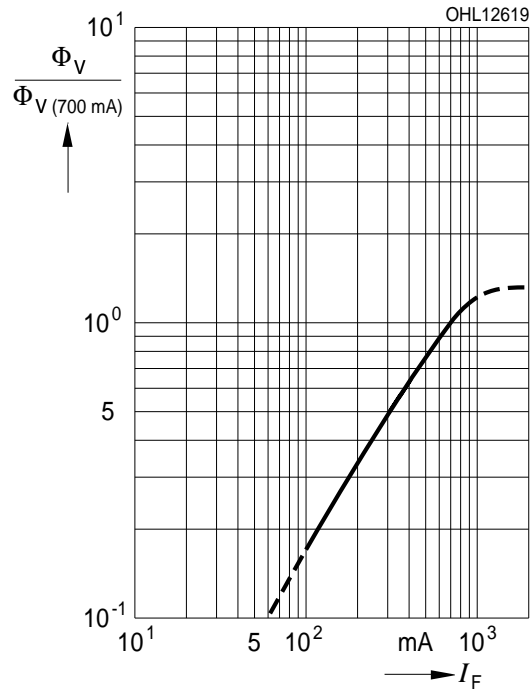
Relativer Lichtstrom 2) Seite 17 Relative Luminous Flux 2) page 17
