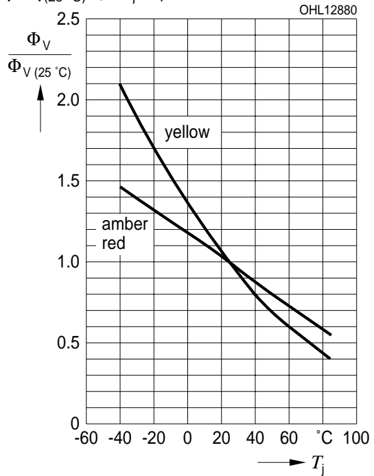
Relativer Lichtstrom 2) Seite 17 Relative Luminous Flux 2) page 17
