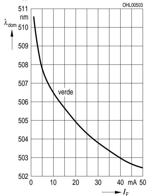
Dominante Wellenlänge \lambda_{\text{dom}} = f(I_F) Dominant Wavelength LV, T_A = 25\text{ °C}
