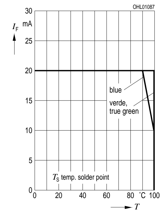
Maximal zulässiger Durchlassstrom I_F = f(T) Max. Permissible Forward Current
