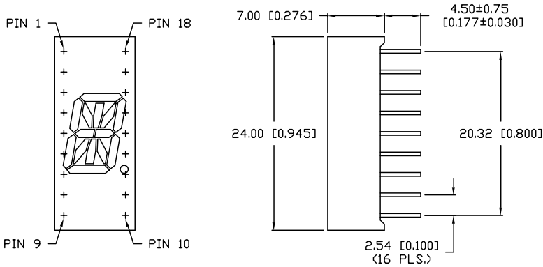
DIGIT DETAIL
