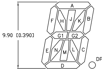
DIGIT DETAIL
