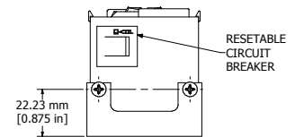
VIEW A-A
