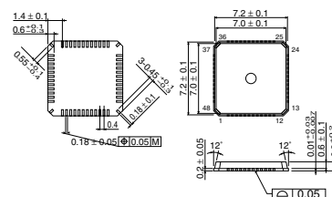
QFN48U
