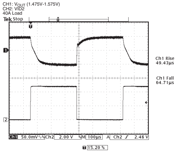
DYNAMIC VID CHANGE
