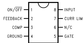
Surface Mount Mini SO-8 Package
