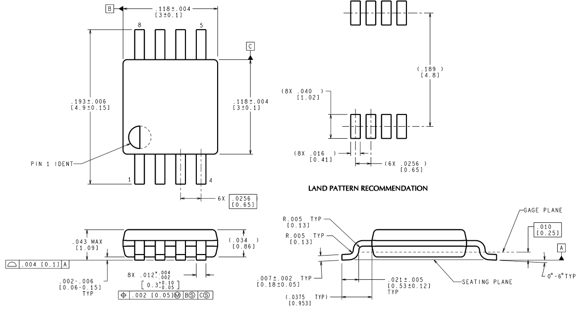
Surface Mount Mini SO-8 Package NS Package Number MUA08A
