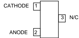
LM4041_F (SOT23)
