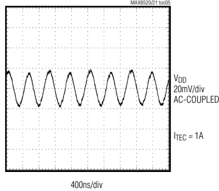
V_{DD} RIPPLE
