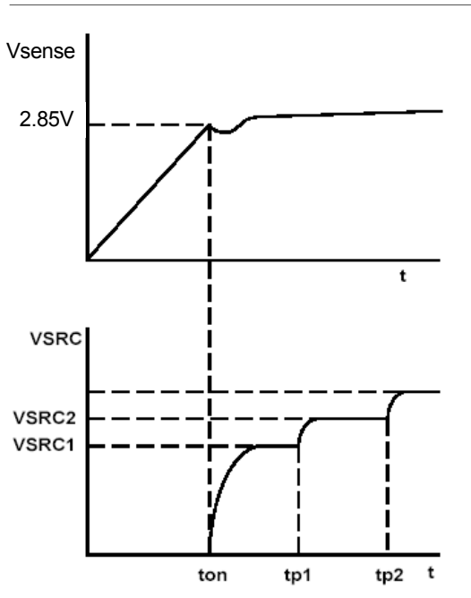
Figure 19 Softstart Phase
