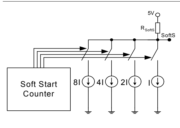
Figure 20 Softstart Circuit
