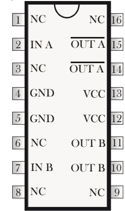
16 Pin SOIC IXDF402SI-16
