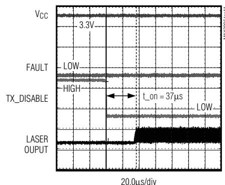
TRANSMITTER ENABLE
