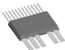
X026a ISOPLUS-DIL™ Weight = 25 g
