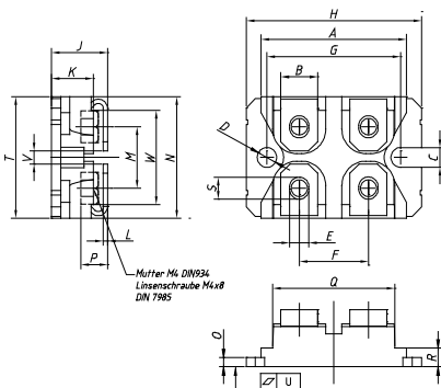
X027a SOT-227 B miniBLOC X027b SOT-227 UI miniBLOC
