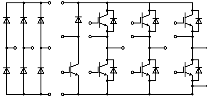
Rectifier
