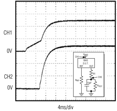
STARTUP DELAY ( V_{BIAS} = 5\text{V} , I_{REF} = 2.5\text{mA} )
