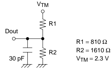
Fig.2 : Output load
