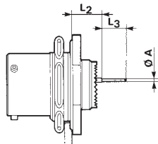
receptacle type 7
