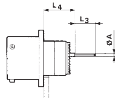
receptacle type 0
