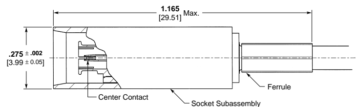
Socket
