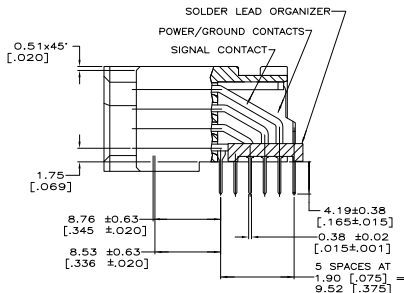
SECTION A-A SCALE 4:1
