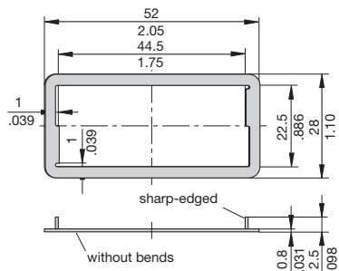
Spacer Y 303 676 01
