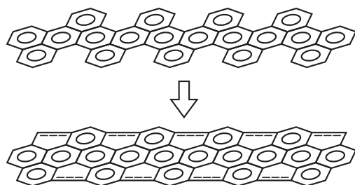
Molecular structure of PAS
