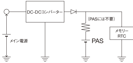
○適用1: 携帯電話
