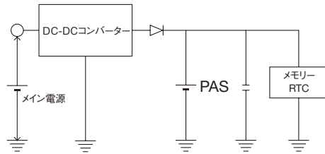
○適用3: 携帯電話
