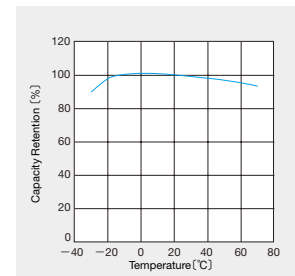
○温度特性 Temperature characteristics
